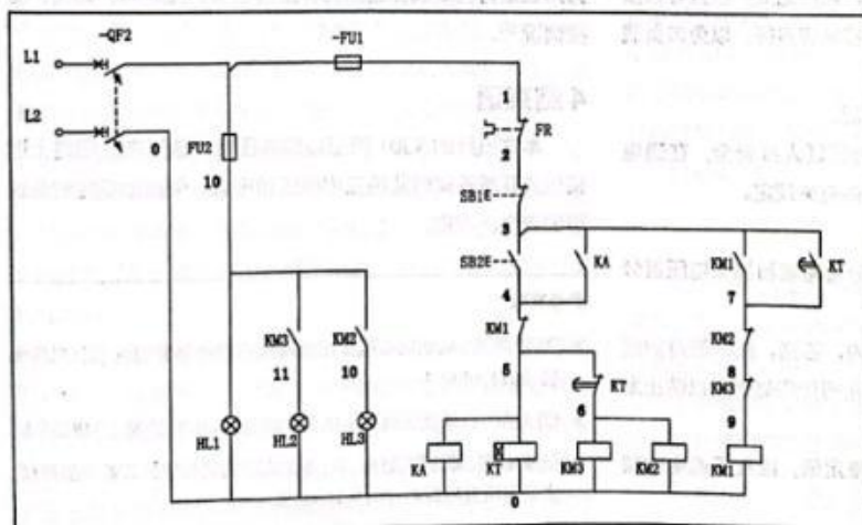
图5 控制回路电路图
