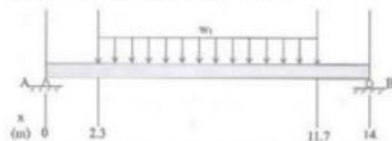
图12 载重臂的纵向截面载荷受力图
