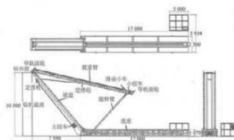
图 1 深井钻机钻杆自动传送装置的机械结构视图
