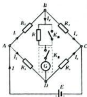
图1 单臂电桥原理图
